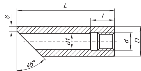
Рис. 4 Бобышка 710-04
