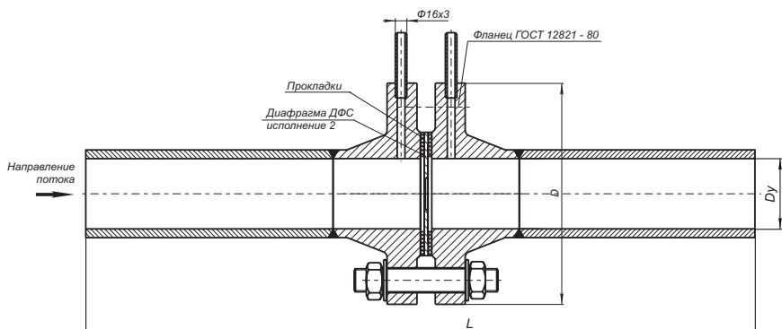
Фланцевое соединение дл.: ДФС
