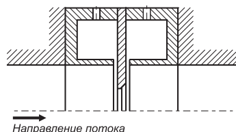
Угловой с кольцевыми щелями
