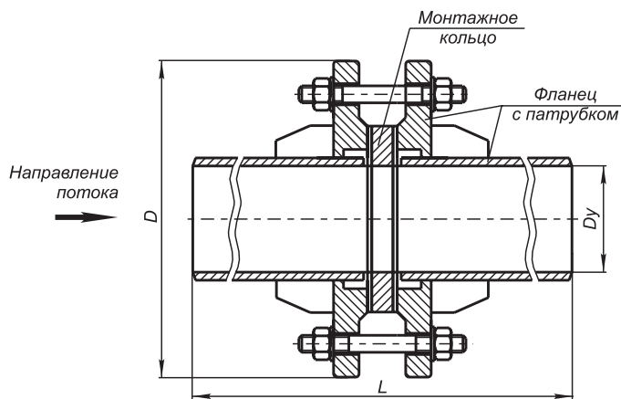
Фланцевое соединение для ДКС. Pу до 0,6...2,5 МПа
